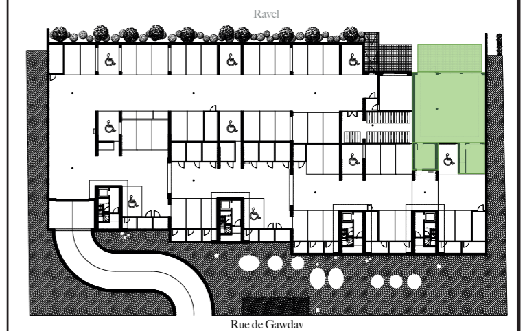
PLAN GENERAL :
