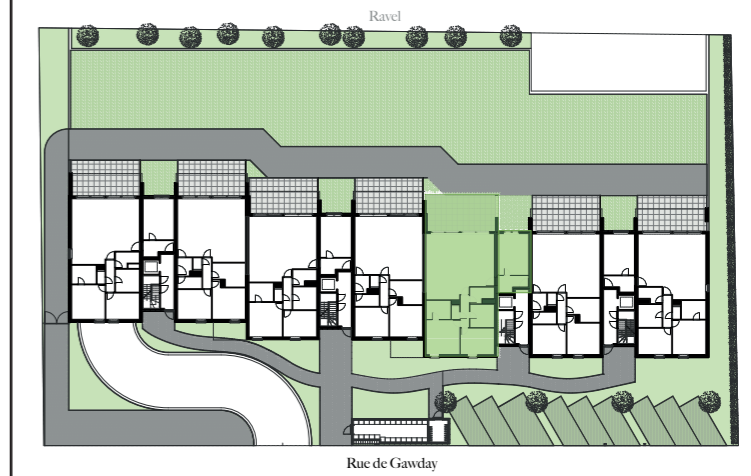
PLAN GENERAL :
